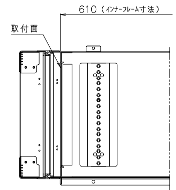
断面A-A
