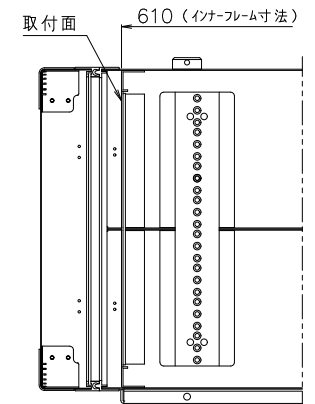
断面A-A
