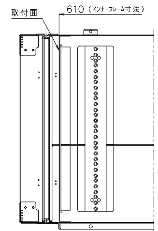
断面A-A
