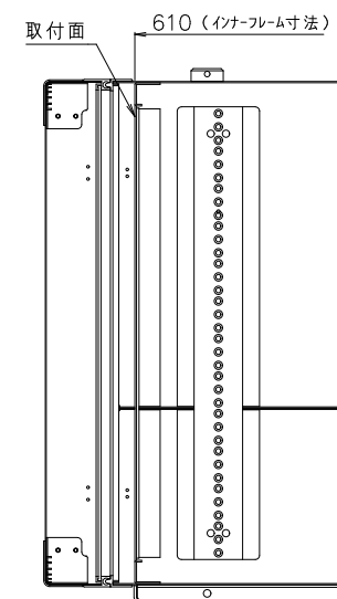
断面A-A
